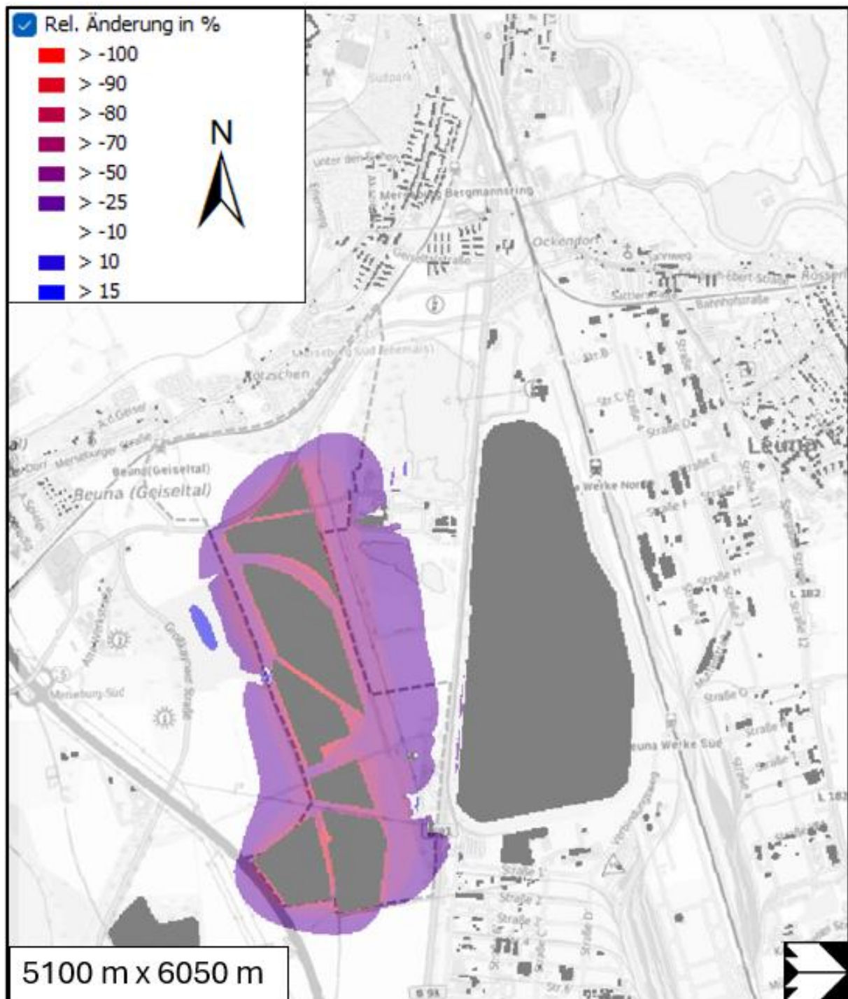
Abb. 7.3: Relative Änderung der jahresmittleren Windgeschwindigkeit im zu betrachtenden Untersuchungsgebiet in 10 m über Grund zwischen Planfall und Istzustand. Plan- gebiet grau gestrichelt hinterlegt. Datenquellen: http://sg.geodatenzentrum.de/web_public/Datenquellen_TopPlus_Open.pdf
